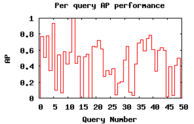
(d) PRF run. Standard deviation: 0.2568
