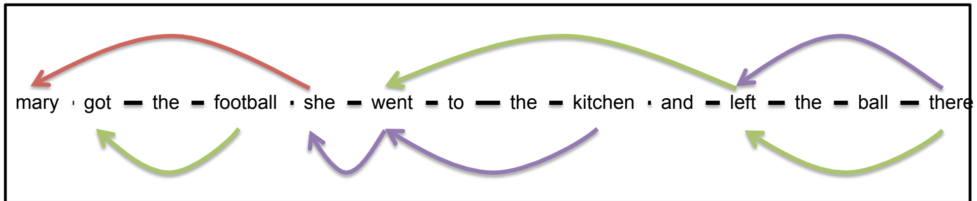
Backward DAG
