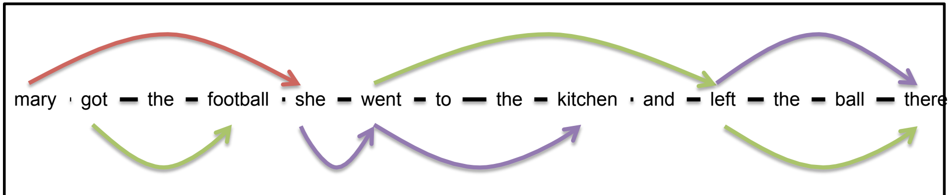
Forward DAG
