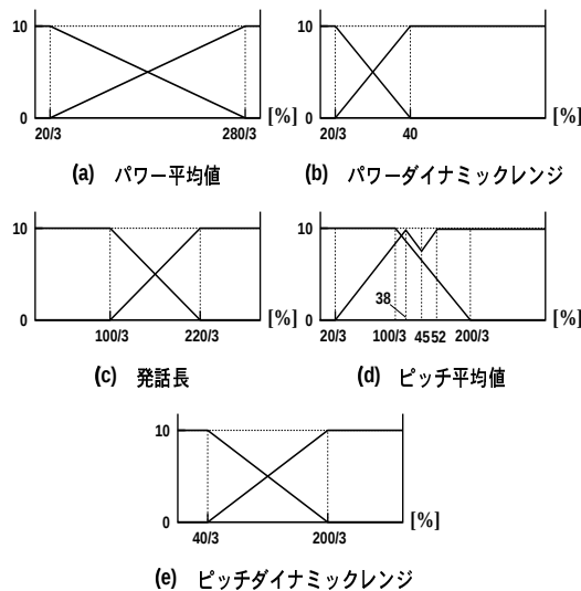
図5 入力メンバーシップ関数
