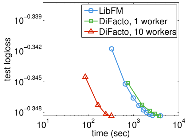
(a) Criteo1
