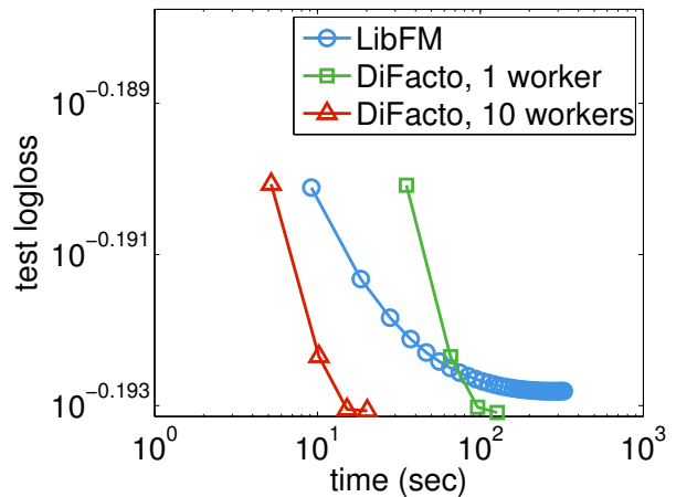
(b) CTR1
