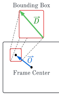
Fig. 23: \vec{O} & \vec{D}
