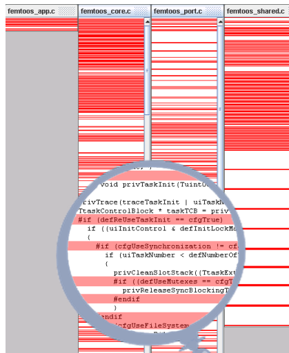
Abbildung 4: Präprozessoranweisungen in Femto OS (rote Linie = Präprozessoranweisung, weiße Linien = C-Code).
