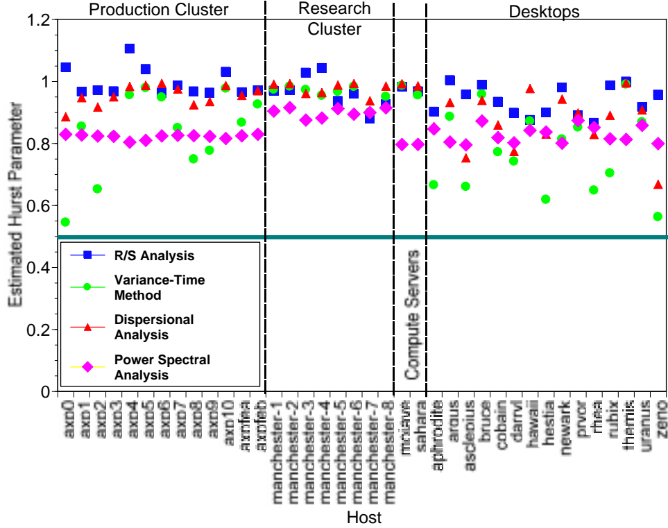
Figure 5: Hurst parameter estimates.
