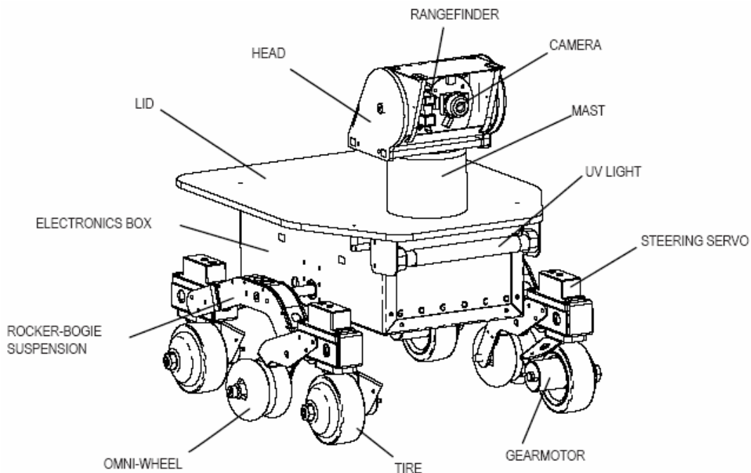
Fig. 2. PER chassis.
