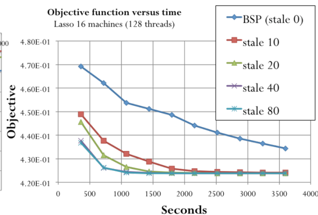
LASSO
