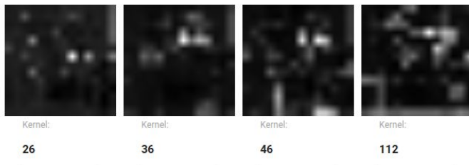
Convolutional Layer : 4
