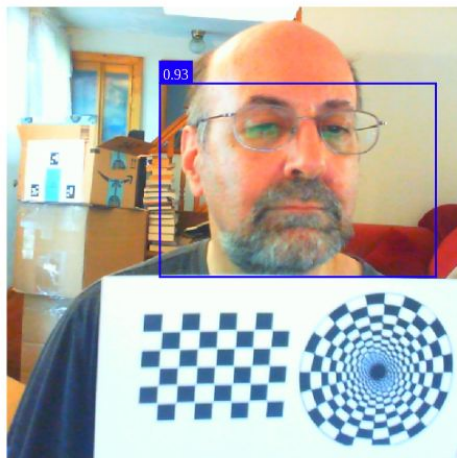
Convolutional Layer : 4
